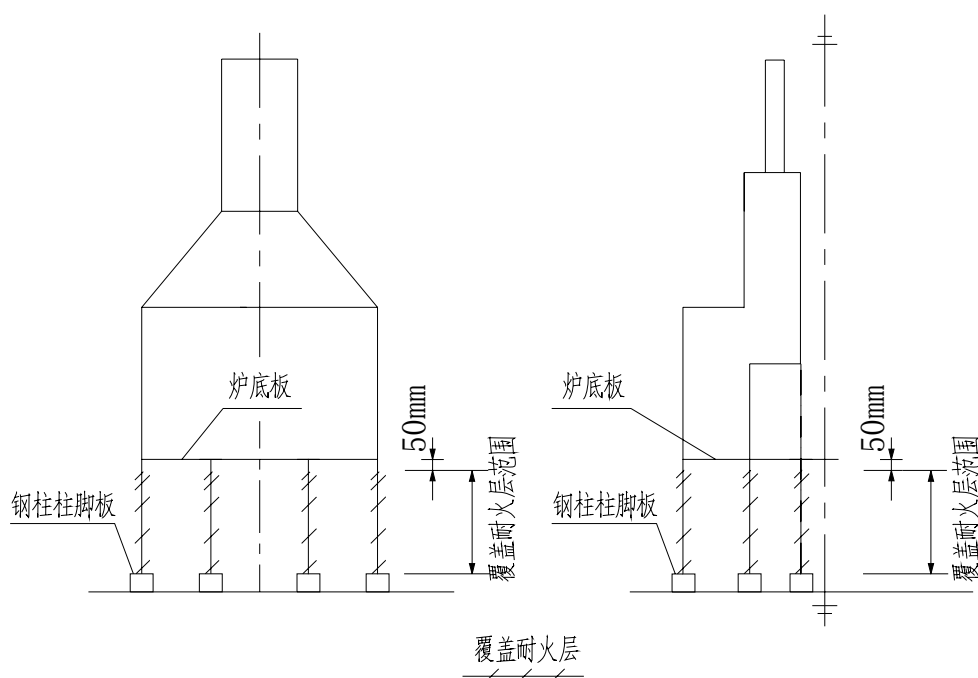
图9 加热炉及乙烯裂解炉
