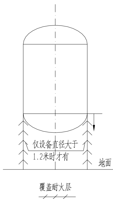
图 5 钢裙座
