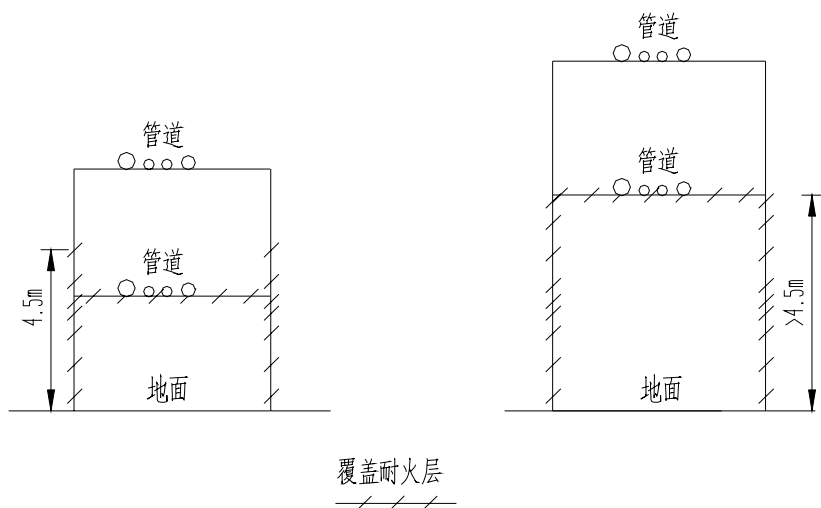
图 6 钢管架 I
