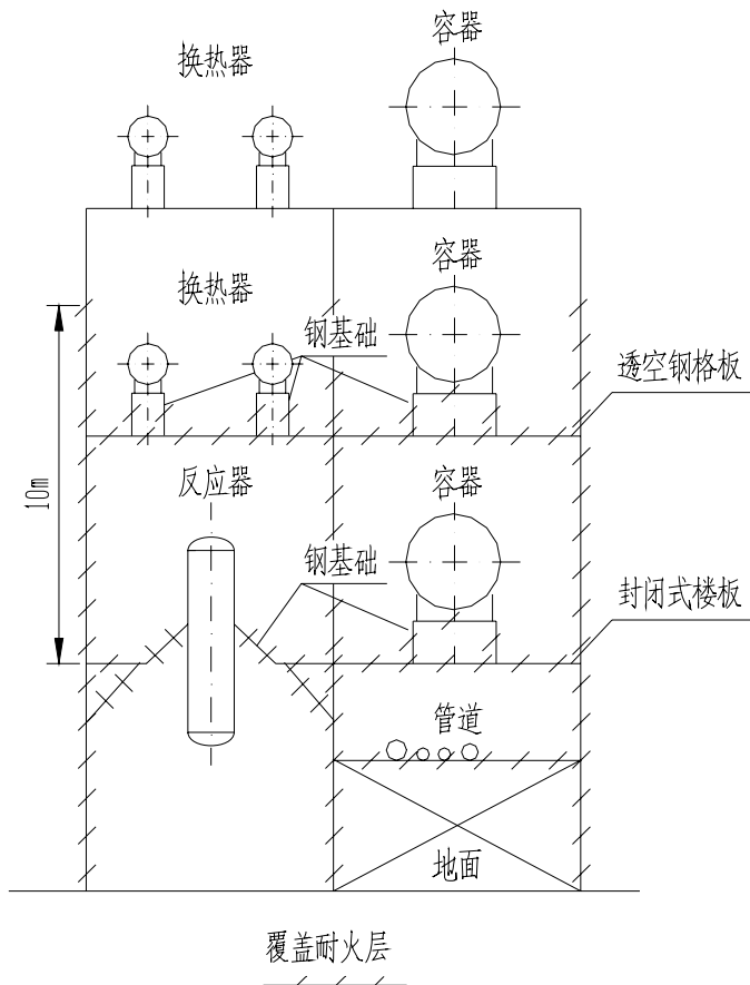
图 4 支承设备钢支架
