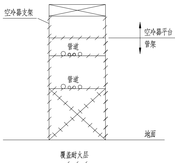
图7 钢管架II
