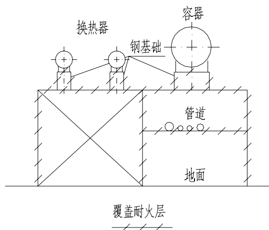
图1 单层构架
