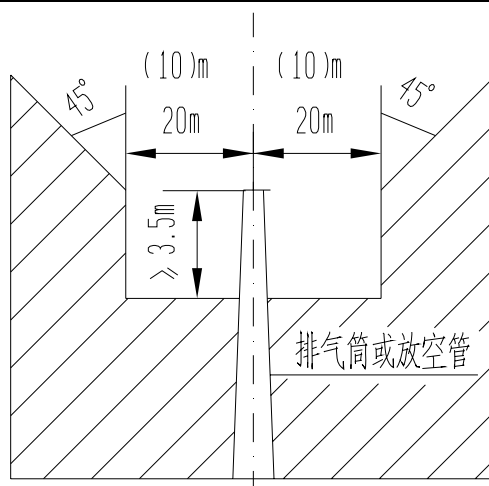
图 5.5.11 可燃气体排气筒、放空管高度示意图
