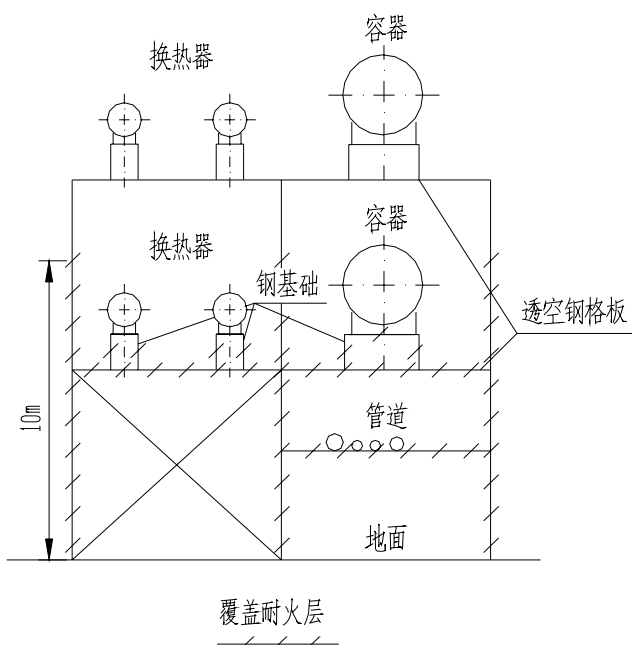
图2 多层构架(楼板为透空的钢格板)
