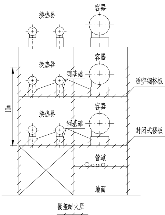
图 3 多层构架 (楼板为封闭式楼板)
